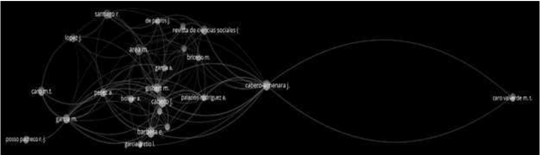
Figura 3: Autores por citación en los documentos
