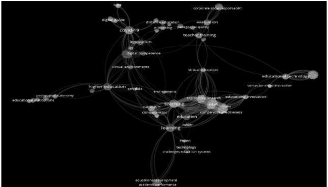
Figura 2: Relaciones de coocurrencia en los nodos
